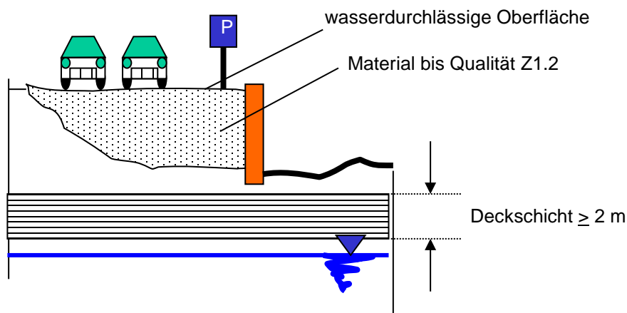
Abbildung 5-3: Z1.2 - Verwertung in technischen Bauwerken ohne definierte technische Sicherheitsmaßnahmen, jedoch bei günstigen hydrogeologischen Verhältnissen
