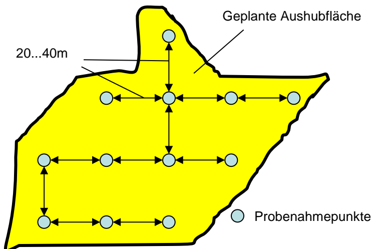
Abbildung 4-2: Rasterabstände
