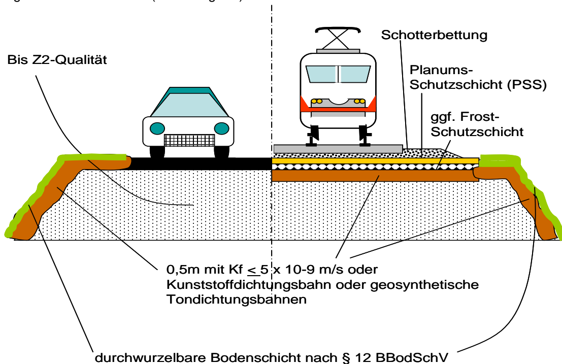
Abbildung 5-7 Regelbauweise Verkehrswegedamm
