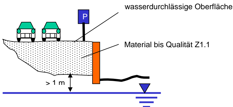
Abbildung 5-2: Z1.1 - Verwertung in technischen Bauwerken ohne definierte technische Sicherungsmaßnahmen
