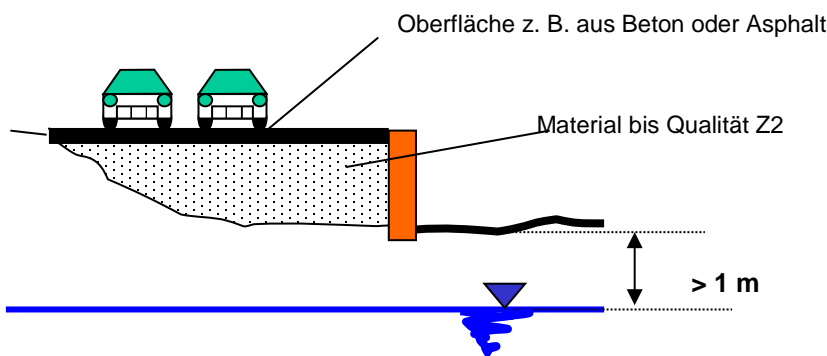
Abbildung 5-4: Z2 - Verwertung in Erdbauwerken ohne bestimmte Geometrie unter einer wasserundurchlässigen Deckschicht (z. B. Oberfläche aus Beton oder Asphalt)
