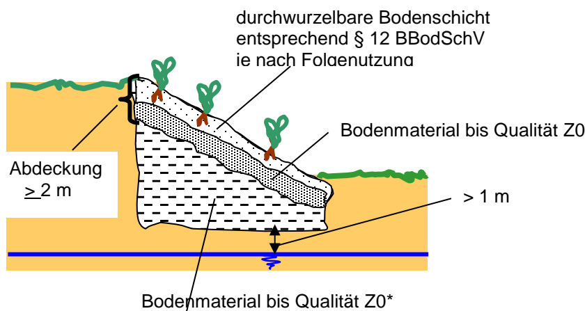
Abbildung 5-1: Z0 und Z0*- Verwertung bei der Verfüllung von Abgrabungen
